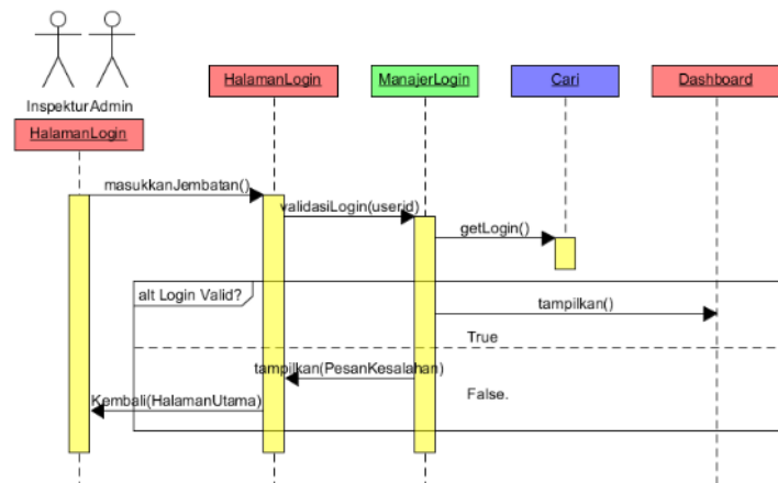
Gambar 5. Sequence Diagram SIG Melakukan Login
