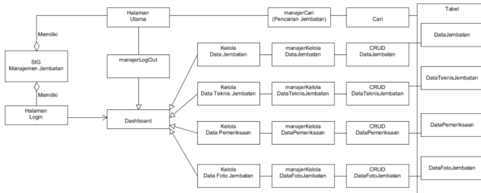
Gambar 6. Class Diagram SIG Manajemen Jembatan Kabupaten Brebes
