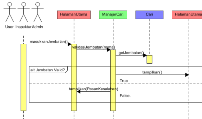
Gambar 4. Sequence Diagram Mencari Informasi Jembatan
