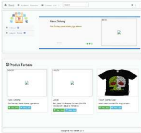
Fig. 7. Main Page
